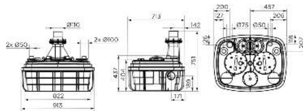
Размеры (мм)
